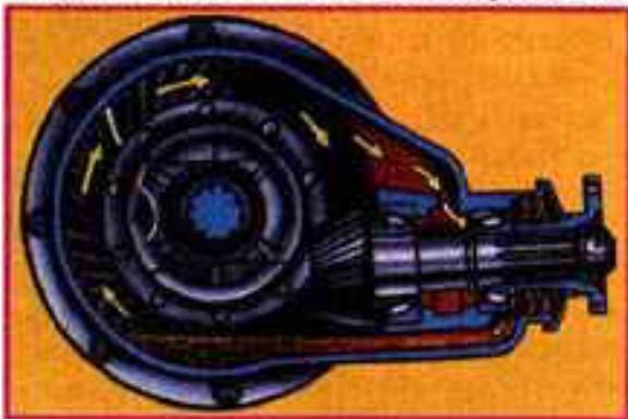
Схема смазки главной передачи
