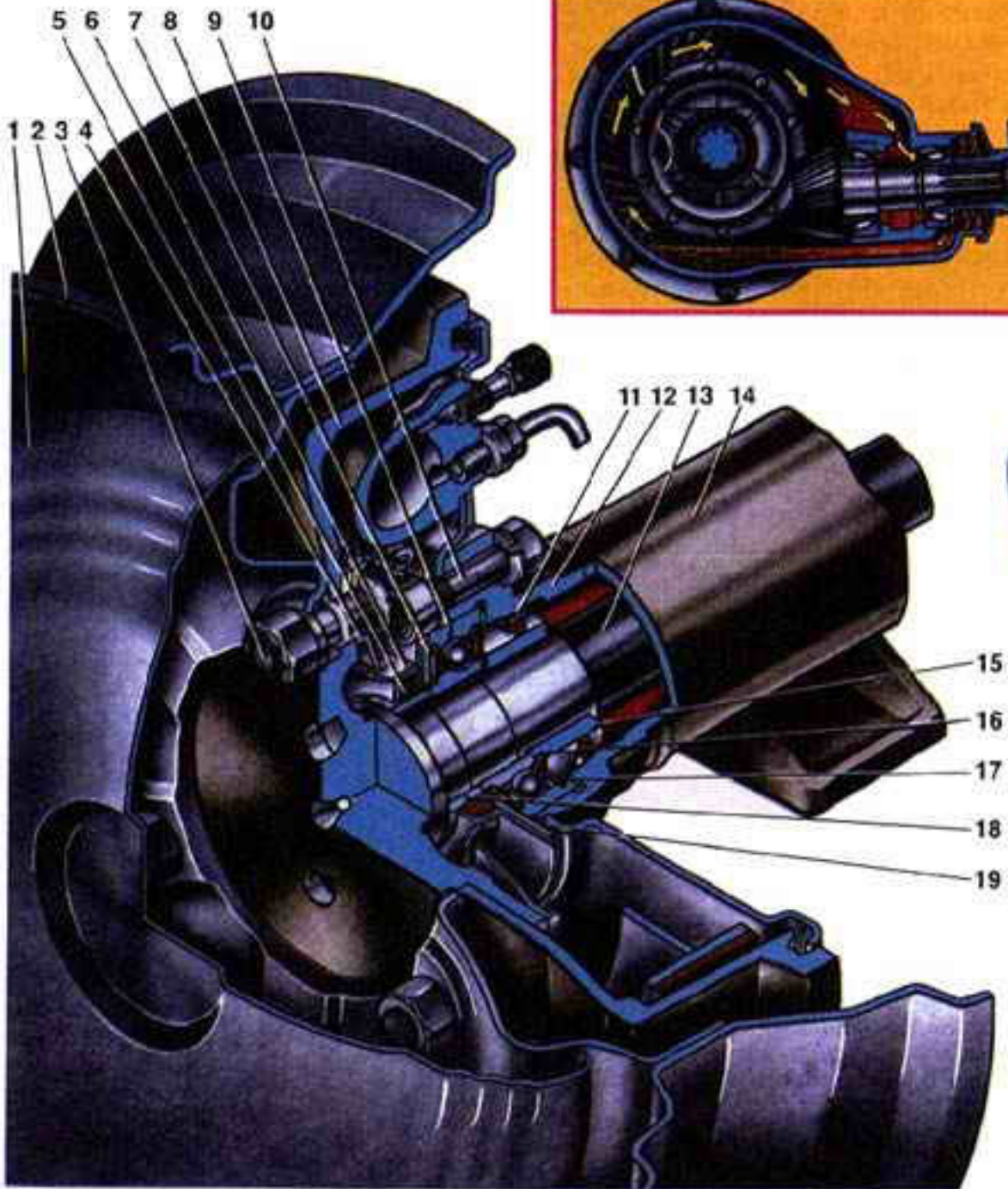
Схема смазки главной передачи
