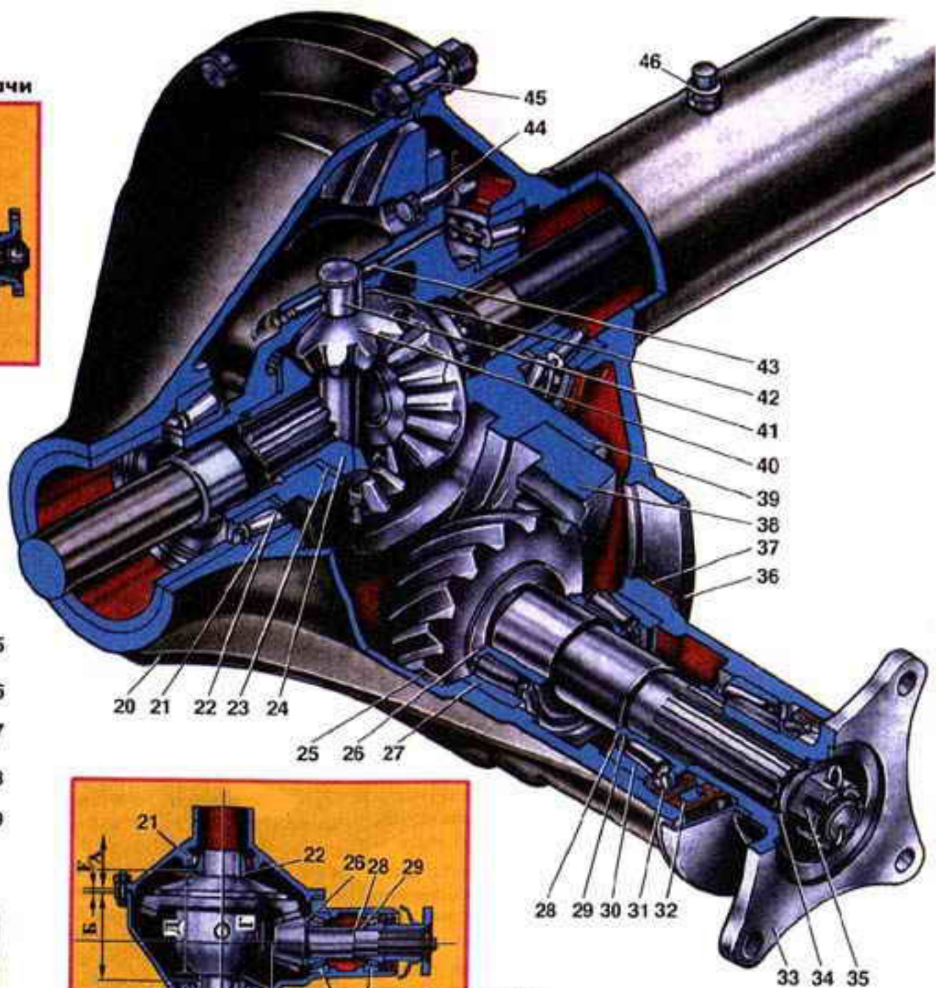
Схема главной передачи
