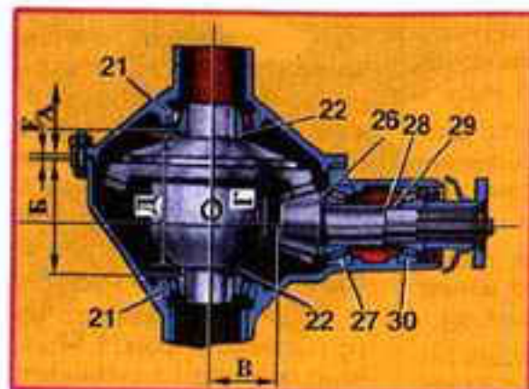
Схема главной передачи
