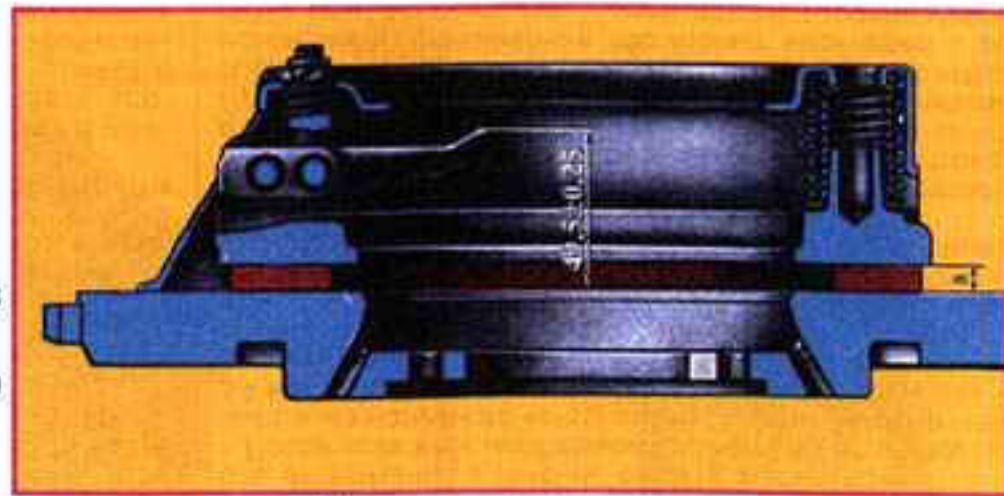
Регулировка сцепления
